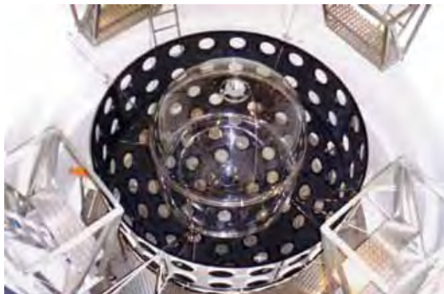
Детектор «Шооз-1»
